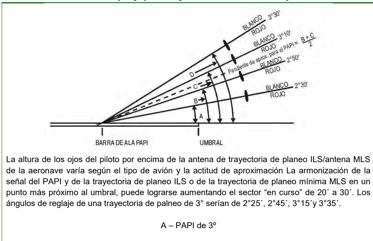
Figura E-20 Haces luminosos y reglaje del ángulo de elevación del PAPI y del APAPI
