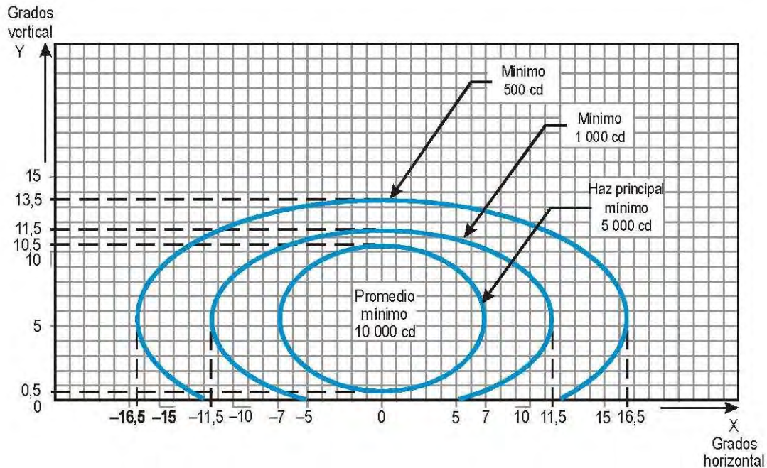
Diagrama de isocandelas para las luces de barra de ala de umbral (luz verde)
