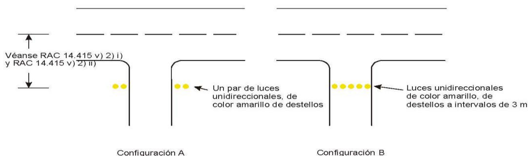
Figura E-29. Luces de protección de pista
