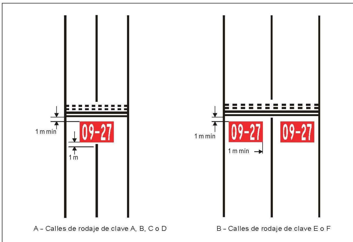
Figura E-10 Señal con instrucciones obligatorias
