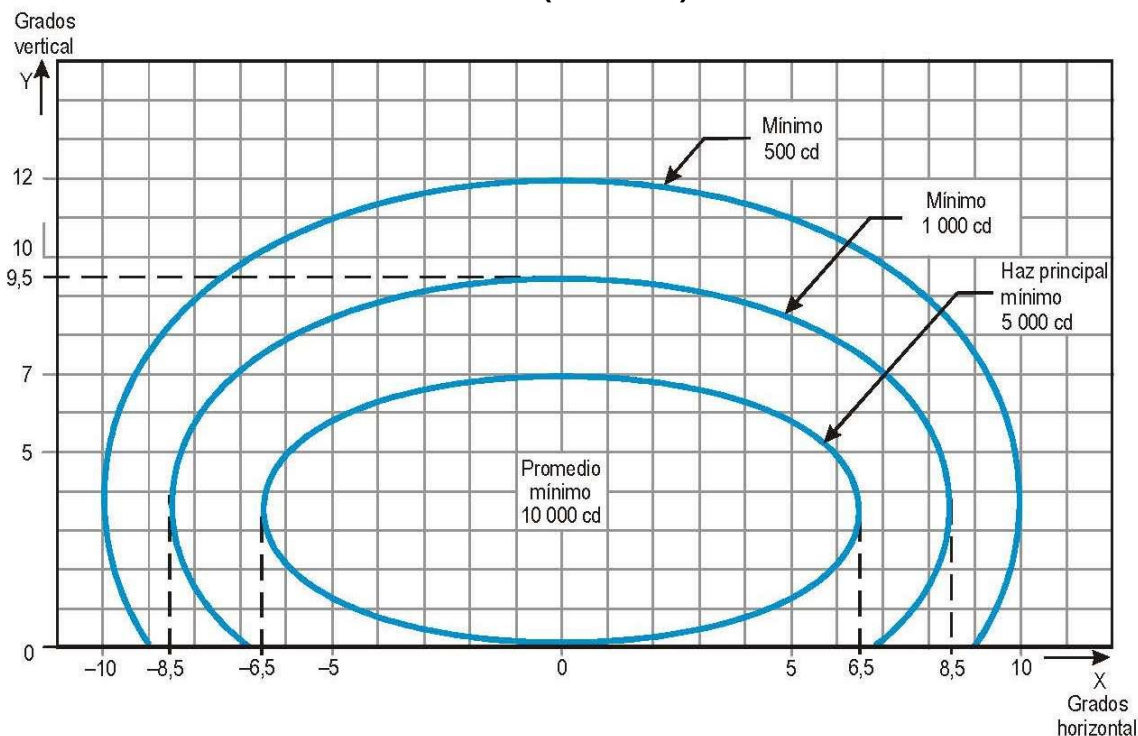
Figura A2-10. Diagrama de isocandelas para las luces de borde de pista cuando el ancho de la pista es de 60 m (luz blanca)
