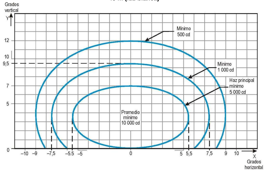
Figura A2-9. Diagrama de isocandelas para las luces de borde de pista cuando el ancho de la pista es de 45 m (luz blanca)
