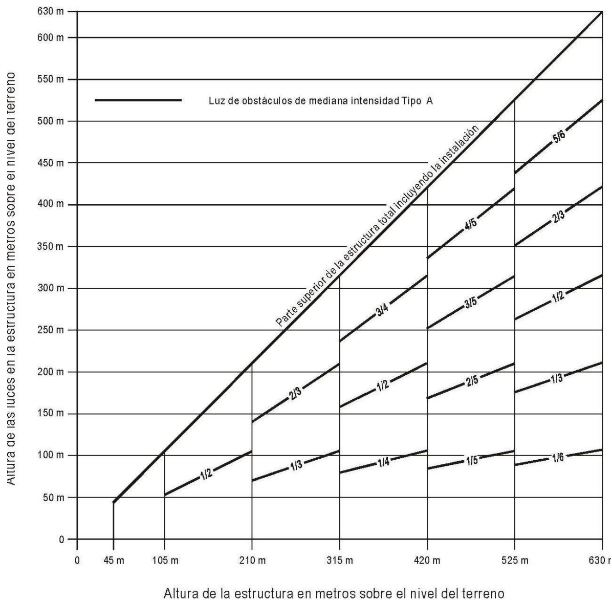
Figura A6-1. Sistema de iluminación de obstáculos con luces blancas de destellos de mediana intensidad de Tipo A
