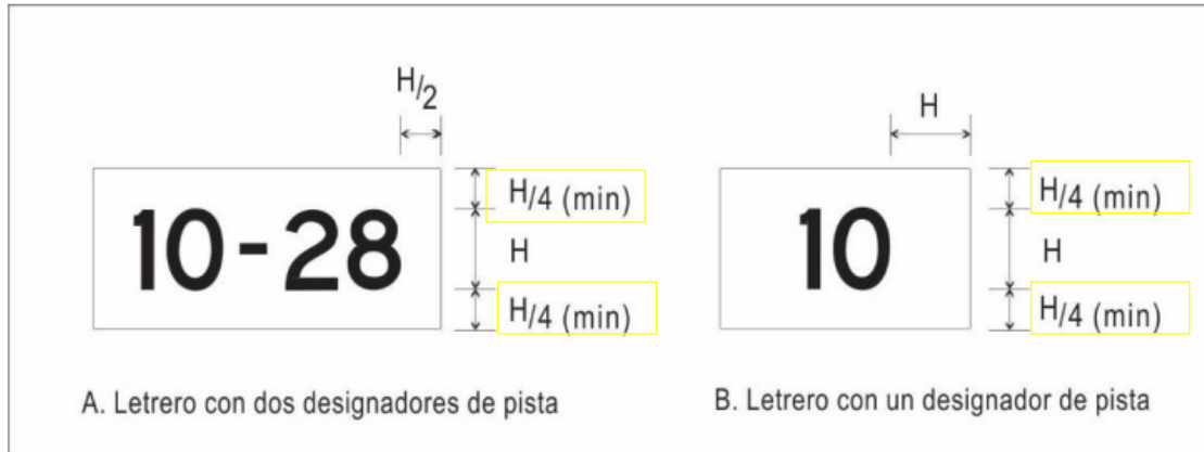
Figura A4-4. Dimensiones de letreros
