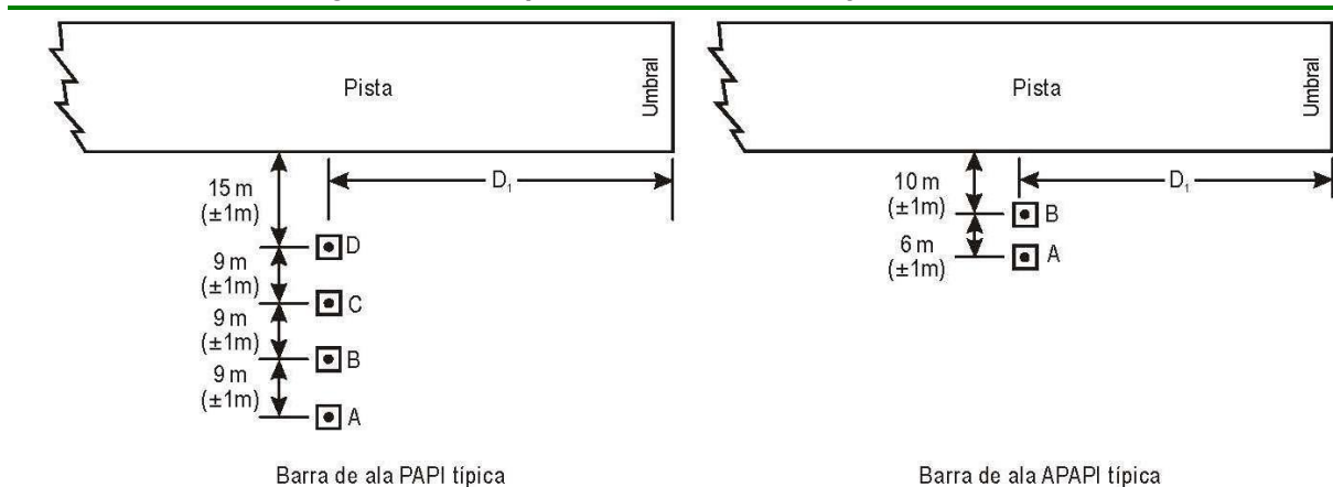
Figura E-19. Emplazamientos del PAPI y del APAPI
