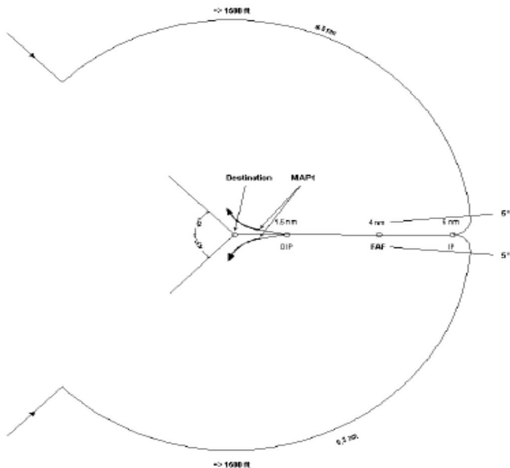
FIGURA 1 Procedimiento del arco
