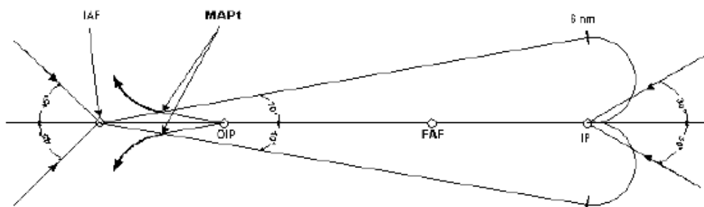
FIGURA 2 Procedimiento de viraje a base y aproximación directa
