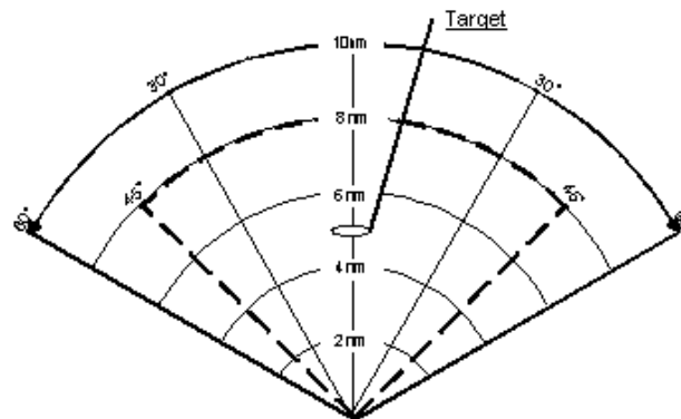
FIGURA 5 Área de aproximación frustrada hacia la izquierda o la derecha
