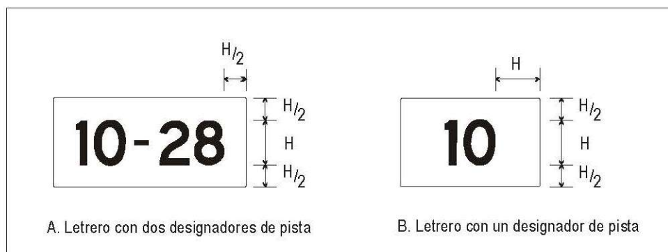
Figura A4-3. Dimensiones de letreros
