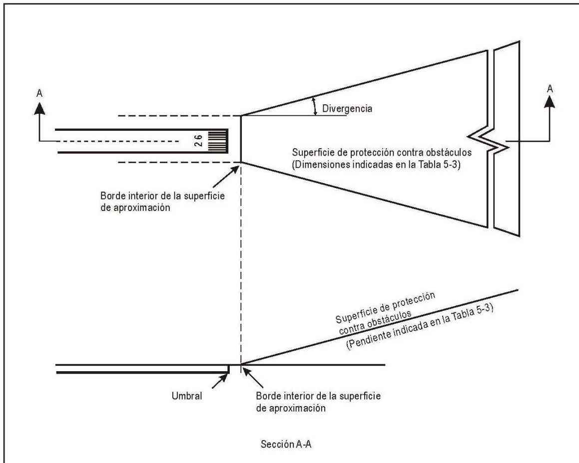
Figura E-21 Superficie de protección contra obstáculos para los sistemas visuales indicadores de pendiente de aproximación
