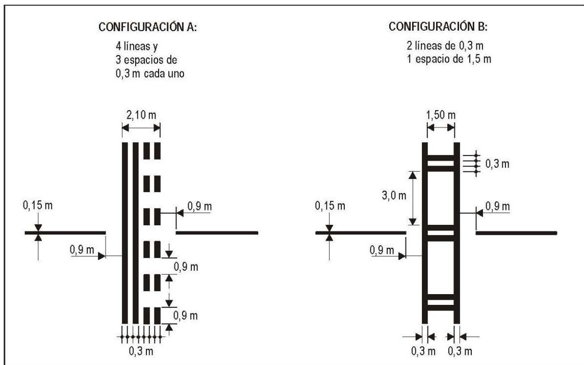
Figura E-8 Señales de punto de espera de la pista
