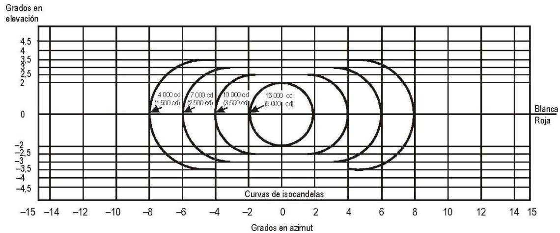
Figura A2-23. Distribución de la intensidad luminosa del PAPI y del APAPI
