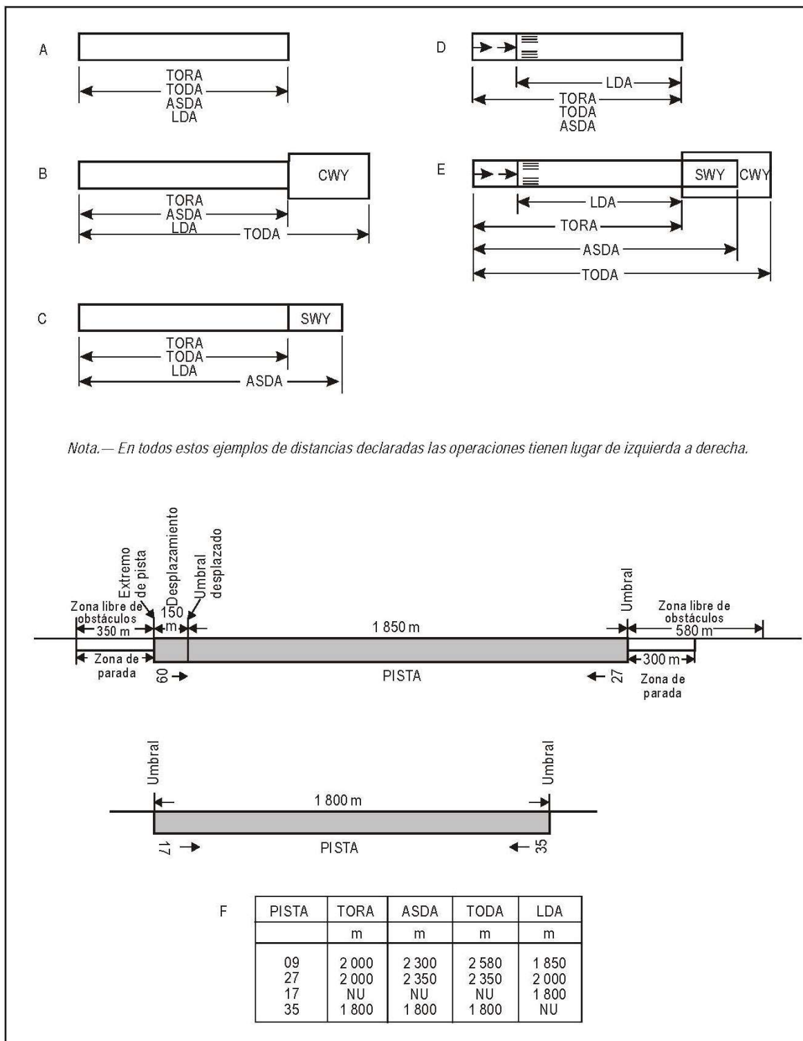
Figura An-1. Distancias declaradas
