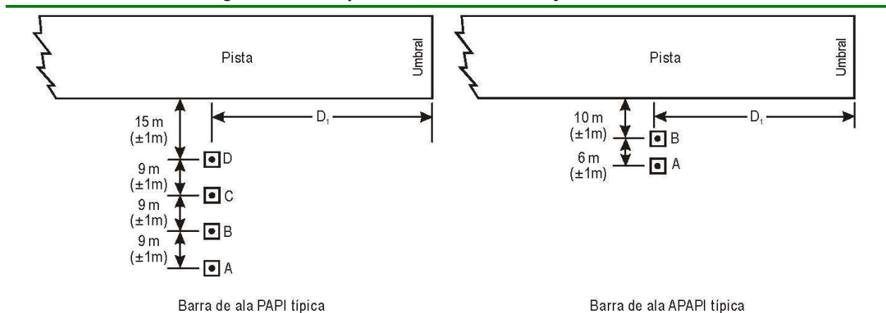
Figura E-19. Emplazamientos del PAPI y del APAPI
