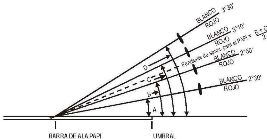
Figura E-20 Haces luminosos y reglaje del ángulo de elevación del PAPI y del APAPI
